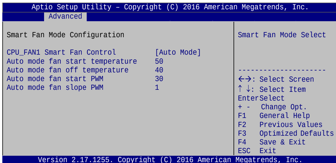
BIOS Menu 10: Smart Fan Mode Configuration
