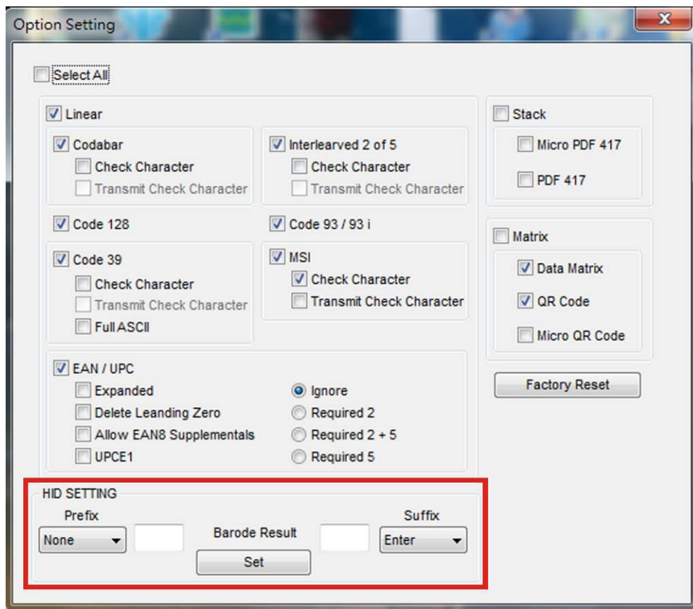
圖表 3-10：Option Setting 選單 – HID 設定
