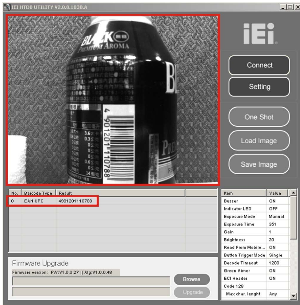
圖表 3-12：主畫面- 載入的影像及資訊
