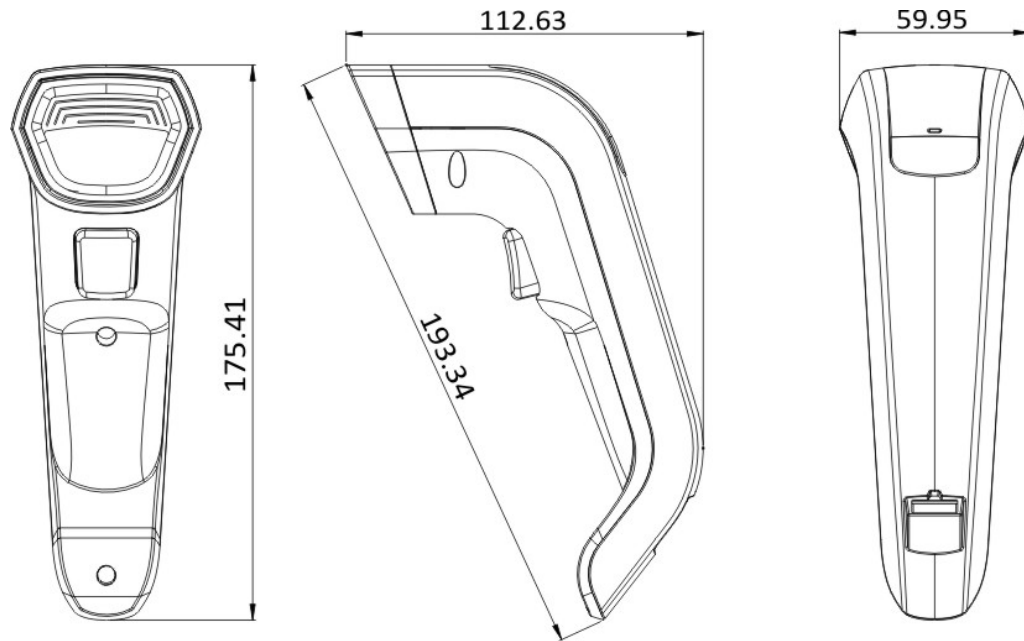
圖表 1-3：尺寸圖（單位：mm）
