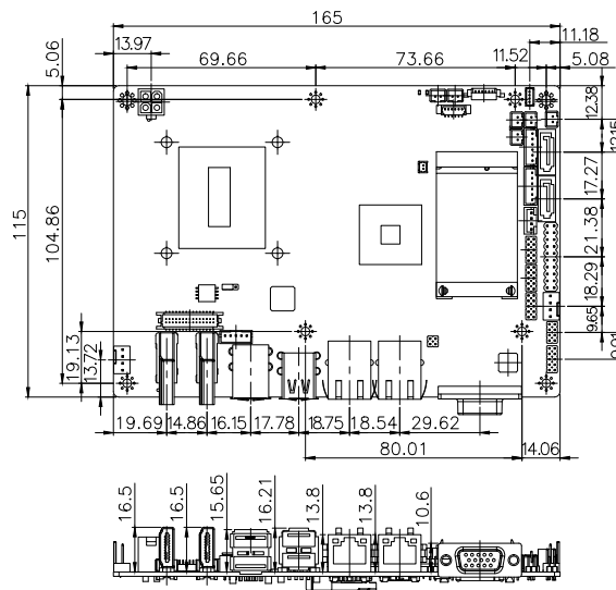
NANO-QM871-i1
