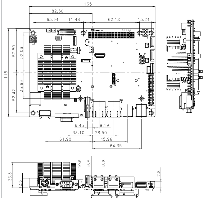
NANO-BTW2/NANO-BT-i1
