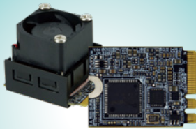
Mustang-M2AE-MX1 Intel® Movidius™ Myriad™ X MA2485 VPU
